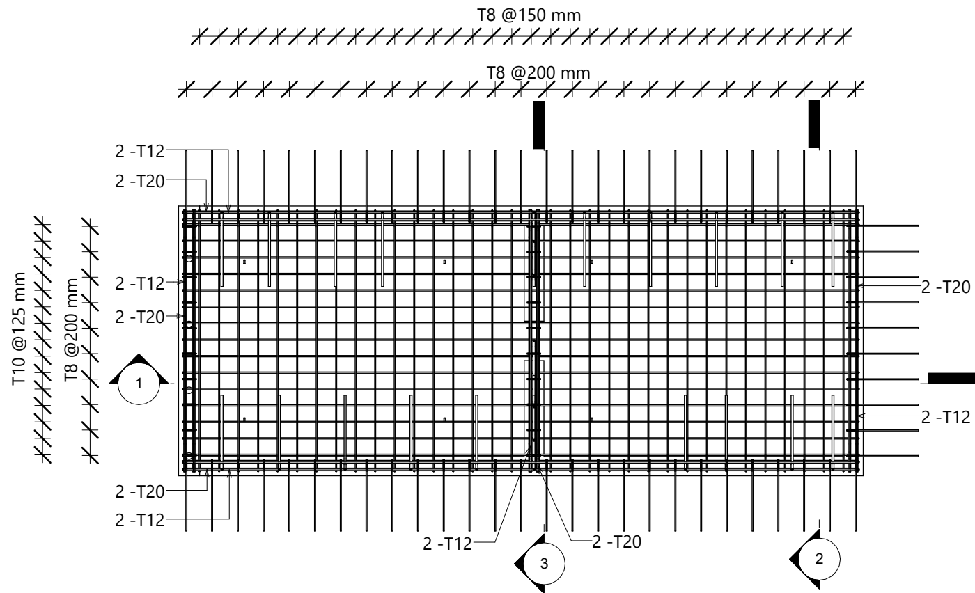
A TOP PLAN(REINF) 1 : 40
