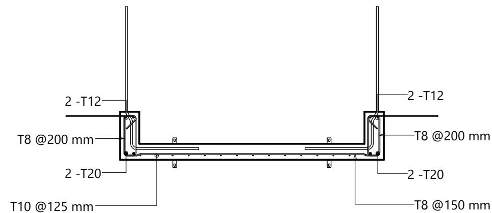
2 SECTION(REINF) 1 : 30
