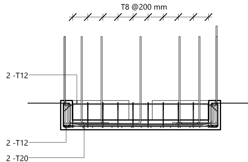
3 SECTION(REINF) 1 : 30
