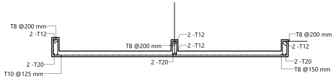
1 SECTION(REINF) 1 : 40
